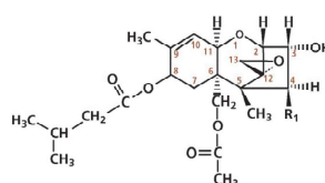
■ Type A-trichothecenes : T-2: (R1=OAc) HT-2 (R1=OH)
